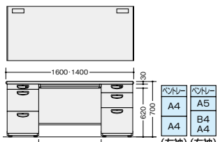
NED167BC-□ NED147BC-□
