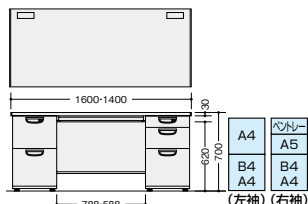
NED167BA-□ NED147BA-□
