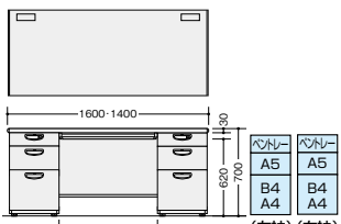
NED167BB-□ NED147BB-□
