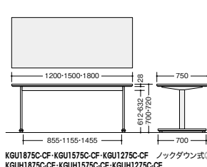
KGU1875C-CF-KGU1575C-CF-KGU1275C-CF ノックダウン式③
