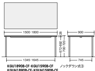
KGU1890B-CF-KGU1590B-CF-KGU1275C-CF ノックダウン式③
