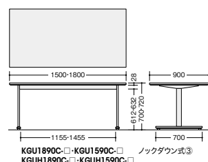
KGUH1890C-CF-KGUH1590C-CF-KGUH1275C-CF ノックダウン式③
