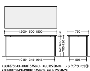
KGU1875B-CF-KGU1575B-CF-KGU1275B-CF ノックダウン式③
