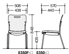
E350F-□ E350-□
