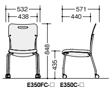
E350FC-□ E350C-□
