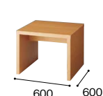
コーナーテーブル TOP PIN ZRT181C-LWA ¥111,600 (受) 外寸法 / W600×D600×H480 天板: メラミン化粧板張りABSエッジ 脚部: PVCシート張り アジャスター付
