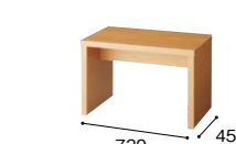
サイドテーブル TOP PIN ZRT181S-LWA ¥110,100 (受) 外寸法 / W730×D450×H480 天板: メラミン化粧板張りABSエッジ 脚部: PVCシート張り アジャスター付
