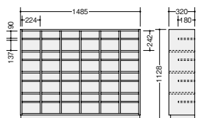
■24人用 SBM-64 ¥315,700 ● 外寸法／W1485×D320×H1128 6列4段 質量：56kg
