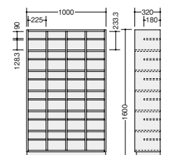
■24人用 SBM-46 ¥270,000 ● 外寸法／W1000×D320×H1600 4列6段 質量：53kg
