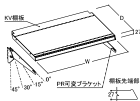
■KV可変棚板セット(W:900mm)
