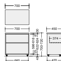
TR074WN-SVZ
