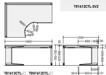
TR1612CTL-□ TRH1612CTL-□
