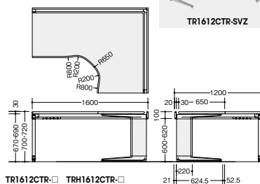
TR1612CTR-□ TRH1612CTR-□
