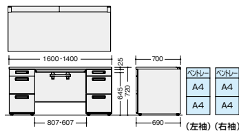
CHD167GG-□ CHD147GG-□
