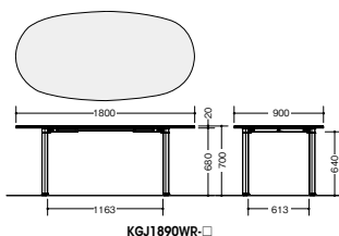
KGJ1890WR-□
