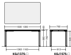
KGJ1375-□ KGJ1575-□
