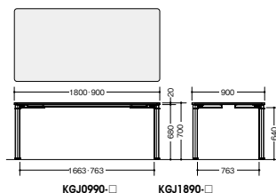
KGJ0990-□ KGJ1890-□
