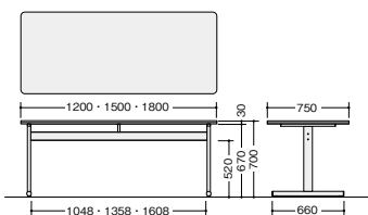
TSN1275-AWH 質量：21kg TSN1875-AWH 質量：27kg
