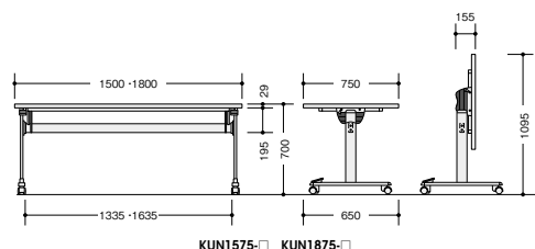
KUN1575-□ KUN1875-□
