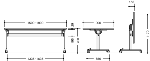
KUN1590-□ KUN1890-□
