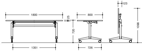
KFN1880-W ¥101,700 ● 外寸法 / W1800×D800×H720 天板: メラミン化粧板張りABS樹脂エッジ 脚部: スチールパイプメラミン焼付塗装仕上 キャスター付 ノックダウン式②
