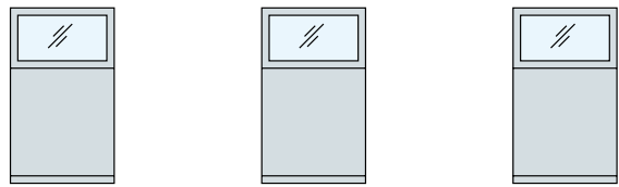
上面ガラス (5mm厚透明ガラス)・下面パネル ❷
