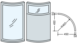
Rガラスパネル (5mm厚透明ガラス) ❷
