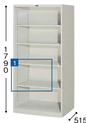
■奥深オープン書庫 KT367-AW ¥68,100○ 外寸法／W880×D515×H1790 棚寸法／W858×D435 内寸法／W830×D513×H1665 付属品：棚板4枚 質量：40kg
