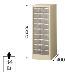
STD109L-B4 ¥41,800 ◆ 外寸法 / W311×D400×H880 引出し内寸法 / W257×D368×H76.8 1列深型9段 / B4縦用 質量: 12.4kg
