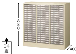
STD318S-B4 ¥128,400 ◆ 外寸法 / W880×D400×H880 引出し内寸法浅型 / W258×D369×H34.5 3列浅型18段 / B4縦用 質量: 35.1kg
