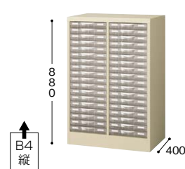
STD218S-B4 ¥90,900 ◆ 外寸法 / W595×D400×H880 引出し内寸法 / W258×D369×H34.5 2列浅型18段 / B4縦用 質量: 24.7kg
