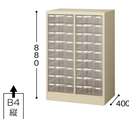
STD209L-B4 ¥70,900 ◆ 外寸法 / W595×D400×H880 引出し内寸法浅型 / W257×D368×H76.8 2列深型9段 / B4縦用 質量: 21.3kg
