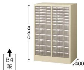
STD266LS-B4 ¥79,800 ◆ 外寸法 / W595×D400×H880 引出し内寸法浅型 / W258×D369×H34.5 引出し内寸法深型 / W257×D368×H76.8 上下コンビ2列 浅型6段・深型6段 / B4縦用 質量: 22.4kg
