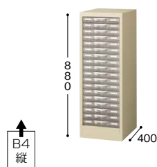
STD118S-B4 ¥51,800 ◆ 外寸法 / W311×D400×H880 引出し内寸法 / W258×D369×H34.5 1列浅型18段 / B4縦用 質量: 14kg
