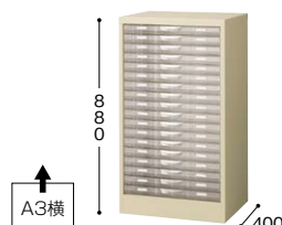
STW118S-A3 ¥62,100 ◆ 外寸法 / W490×D400×H880 引出し内寸法 / W437×D313×H34.4 1列浅型18段 / A3横用 質量: 18.7kg
