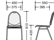
E117-□
