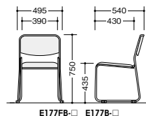
E177FB-□ E177B-□
