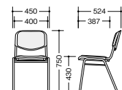
E100-□
