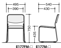
E177FM-□ E177M-□
