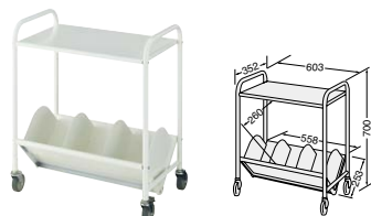
225-30 ¥32,000 外寸法 / W603×D352×H700 付属品: 仕切板4枚付 A4判・B5判用 キャスター付 ノックダウン式 質量: 10.8kg
