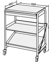
225-17 ¥88,700 外寸法 / W696×D480×H850 引出し有効内寸法 / W596×D393 棚有効寸法 / W620×D400 キャスター付 ノックダウン式 質量: 22.5kg
