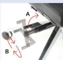
A: ガス上下調整レバー B: ロッキング強度調整レバー
