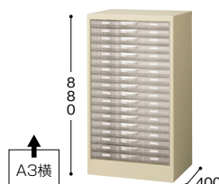
STW118S-A3 ￥67,700◇ 外寸法 / W490×D400×H880 引出し内寸法 / W437×D313×H34.4 1列浅型18段 / A3横用 質量 : 18.7kg
