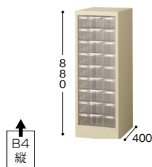
STD109L-B4 ￥45,600◇ 外寸法 / W311×D400×H880 引出し内寸法 / W257×D368×H76.8 1列深型9段 / B4縦用 質量 : 12.4kg
