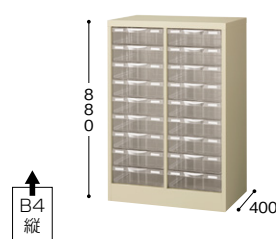
STD209L-B4 ￥77,300◇ 外寸法 / W595×D400×H880 引出し内寸法浅型 / W257×D368×H76.8 2列深型9段 / B4縦用 質量 : 21.3kg
