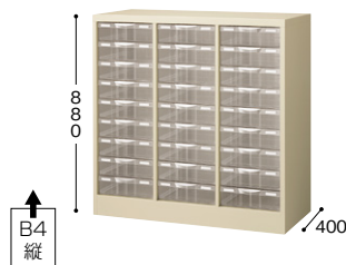
STD309L-B4 ￥106,700◇ 外寸法 / W880×D400×H880 引出し内寸法 / W257×D368×H76.8 3列深型9段 / B4縦用 質量 : 30kg
