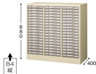
STD318S-B4 ￥140,000◇ 外寸法 / W880×D400×H880 引出し内寸法浅型 / W258×D369×H34.5 3列浅型18段 / B4縦用 質量 : 35.1kg
