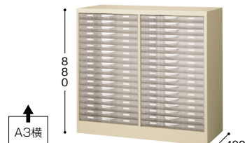
STW218S-A3 ￥127,600◇ 外寸法 / W953×D400×H880 引出し内寸法 / W437×D313×H34.4 2列浅型18段 / A3横用 質量 : 34.1kg
