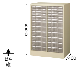
STD266LS-B4 ￥87,000◇ 外寸法 / W595×D400×H880 引出し内寸法浅型 / W258×D369×H34.5 引出し内寸法深型 / W257×D368×H76.8 上下コンビ2列 浅型6段・深型6段 / B4縦用 質量 : 22.4kg
