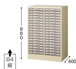
STD218S-B4 ￥99,100◇ 外寸法 / W595×D400×H880 引出し内寸法 / W258×D369×H34.5 2列浅型18段 / B4縦用 質量 : 24.7kg
