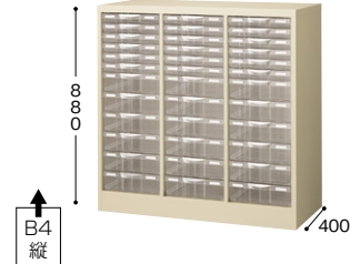
STD366LS-B4 ￥121,400◇ 外寸法 / W880×D400×H880 引出し内寸法浅型 / W258×D369×H34.5 引出し内寸法深型 / W257×D368×H76.8 上下コンビ3列 浅型6段・深型6段 / B4縦用 質量 : 31.7kg
