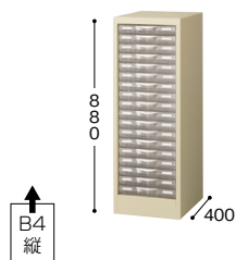
STD118S-B4 ￥56,500◇ 外寸法 / W311×D400×H880 引出し内寸法 / W258×D369×H34.5 1列浅型18段 / B4縦用 質量 : 14kg
