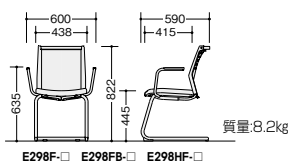
E298F-□ E298FB-□ E298HF-□
