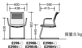
E298-□ E298B-□ E298H-□ E298V-□ E298VB-□ E298HV-□
