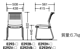
E292-□ E292B-□ E292H-□ E292V-□ E292VB-□ E292HV-□
