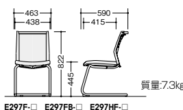
E297F-□ E297FB-□ E297HF-□
