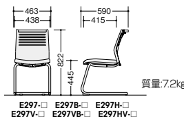
E297-□ E297B-□ E297H-□ E297V-□ E297VB-□ E297HV-□
