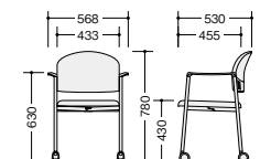
E164FBC-□ E164BC-□
