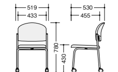
E163FBC-□ E163BC-□
