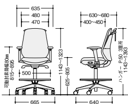
BCE523FAH-□ BCE523FA-□ (ハンガーなし) BCEB523FAH-□ BCEB523FA-□ (ハンガーなし)
