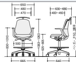
BCE521FH-□ BCE521F-□ (ハンガーなし) BCEB521FH-□ BCEB521F-□ (ハンガーなし) BCE520FH-□ BCE520F-□ (ハンガーなし) BCEB520FH-□ BCEB520F-□ (ハンガーなし)
