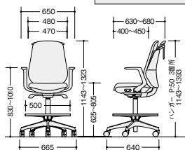
BCE523FH-□ BCE523F-□ (ハンガーなし) BCEB523FH-□ BCEB523F-□ (ハンガーなし) BCE522FH-□ BCE522F-□ (ハンガーなし) BCEB522FH-□ BCEB522F-□ (ハンガーなし)
