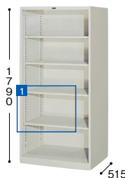
■奥深オープン書庫 KT367-AW ¥84,000○ 外寸法／W880×D515×H1790 棚寸法／W858×D435 内寸法／W830×D513×H1665 付属品：棚板4枚 質量：40kg
