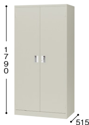
■奥深両開き書庫 K367N-AW ¥103,200○ 外寸法／W880×D515×H1790 棚寸法／W858×D435 内寸法／W810×D483×H1628 付属品：棚板4枚 質量：55kg
