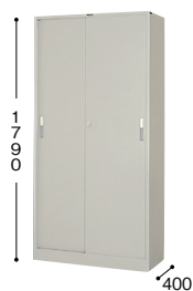
■引違い書庫(スチール戸) HS36J-AW ¥90,000○ 外寸法／W880×D400×H1790 棚寸法／W860×D310 内寸法／W820×D340×H1655 付属品：棚板4枚 質量：51kg
