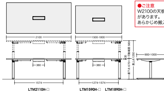
LTM2110H-□
