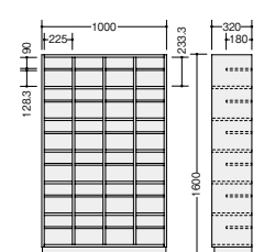
■24人用 SBM-46 ¥315,900 ◆ 外寸法／W1000×D320×H1600 4列6段 質量：53kg
