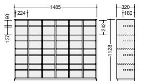
■24人用 SBM-64 ¥366,300 ◆ 外寸法／W1485×D320×H1128 6列4段 質量：56kg
