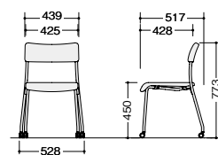
E364FC-□□ 質量:4.1kg
