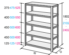
■H型ボード棚 棚板1段の最大積載質量(等分布) 300kg ※W1835×D630タイプは200kg W1535×D630タイプは250kgになります。
